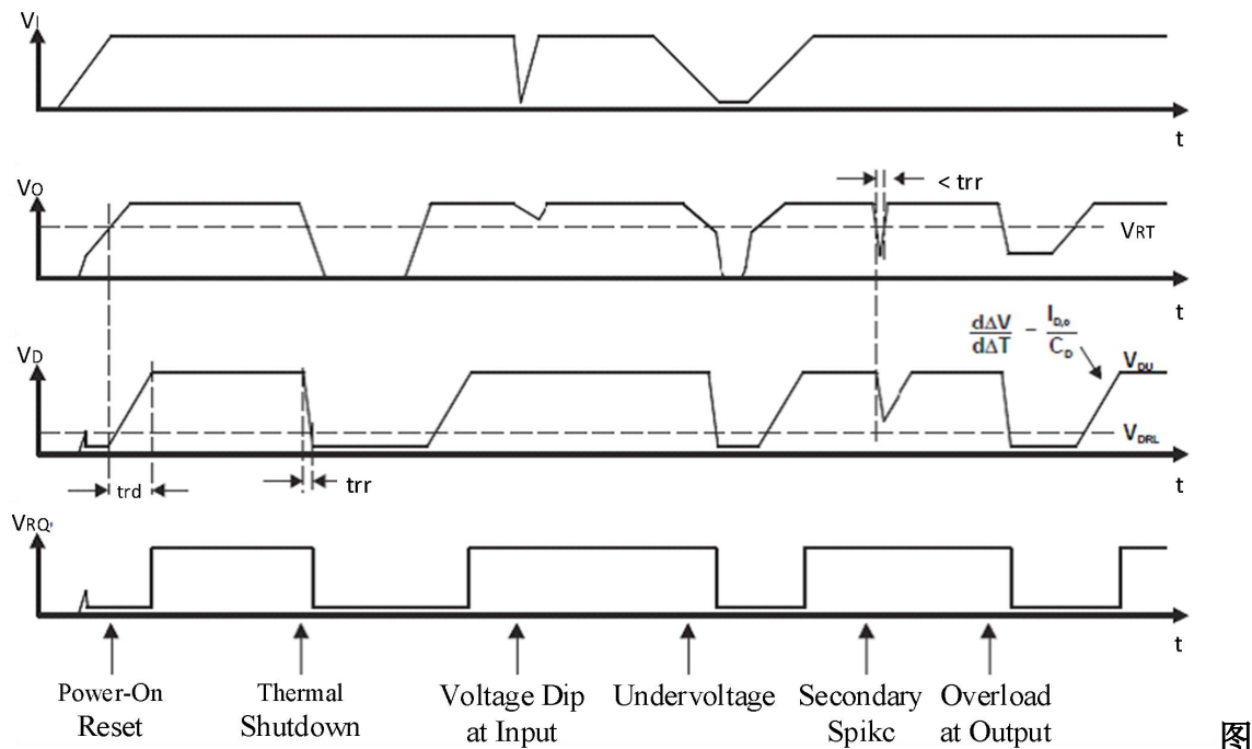
6-1 复位时序
